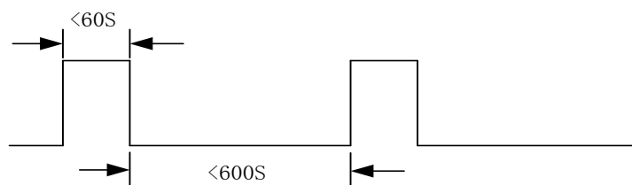
图 3 瞬时脉冲示意图
