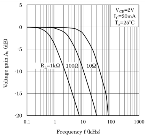
Fig.15 周波数特性
