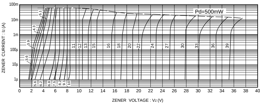
Fig.1 ツェナー特性
