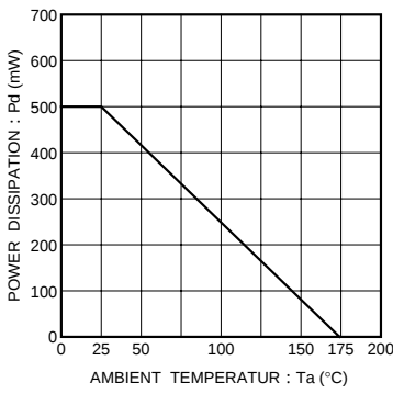
Fig.2 デイレティングカーブ
