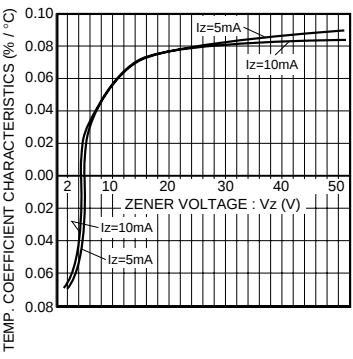
Fig.3 温度系数特性
